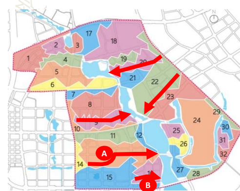
优化后排水分区
