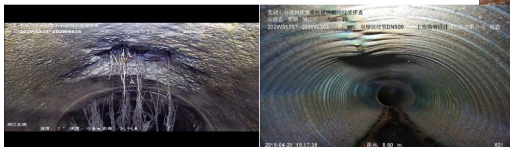
管道结构性缺陷
