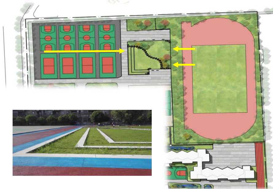
雨水源头减排和排涝除险设施的组合 (池州第十中学海绵改造)
