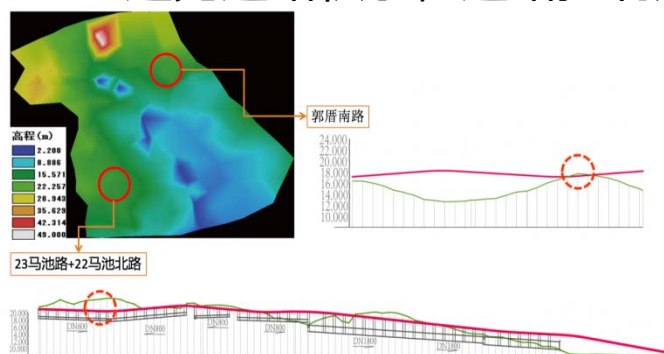
高程分析
